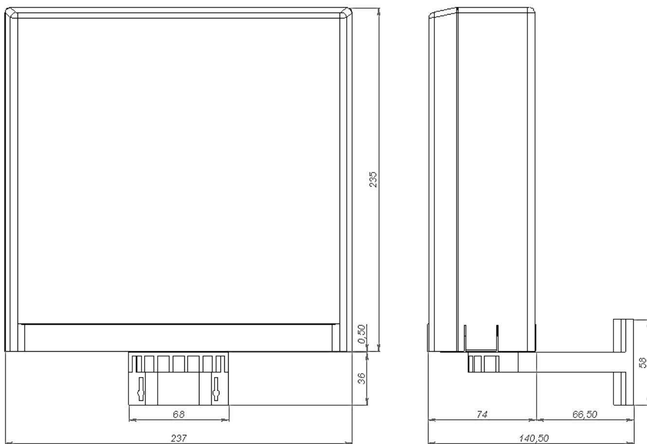
Рис.1 Габаритные размеры VT- BOX15.
